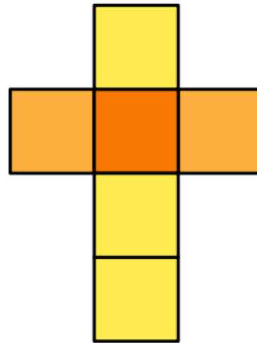
Slika 2: Mreža kocke
